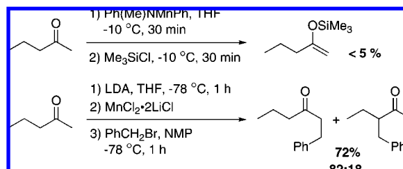
Scheme 158
