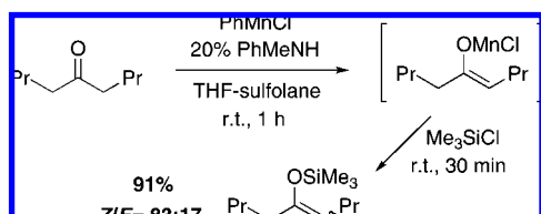
Scheme 145
