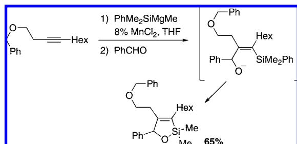
Scheme 221
