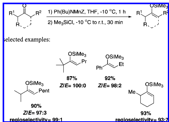
Scheme 145
